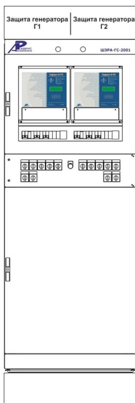
Шкаф защиты генератора (-ов) малой и средней мощности ШЭРА-ГС-2001 БПВА.656457.160, БПВА.650645.001 ТУ
